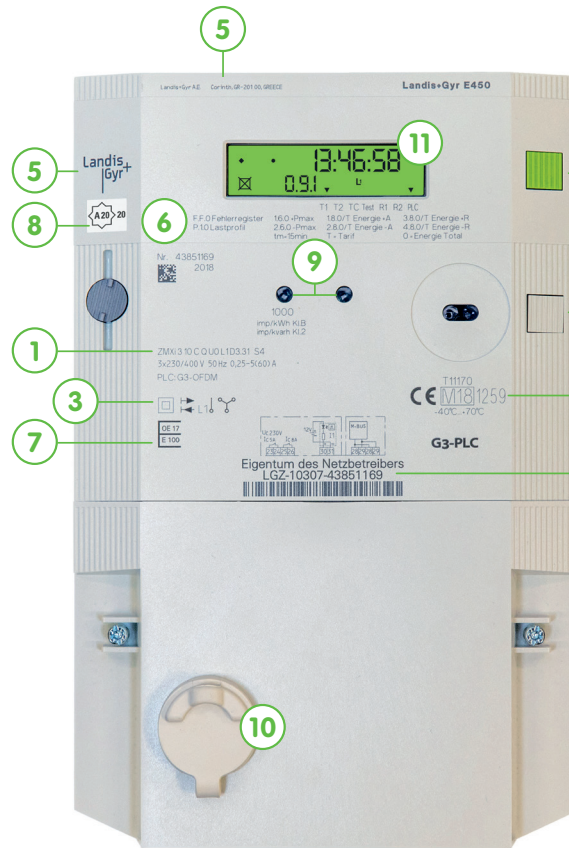
E450 Series 4 G3-PLC 3-ph ZMXi310CQ (Drehstromzähler)
