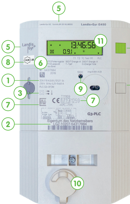
E450 Series 4 G3-PLC 1-ph ZCXi110AQ (Wechselstromzähler)
